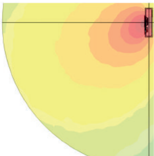
Umgekehrte HF-Horn Position und seine gleichmäßige Abstrahlung
