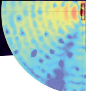
Klassisches Design des HF-Horns auf der Oberseite und seine geriffelte Abstrahlung
